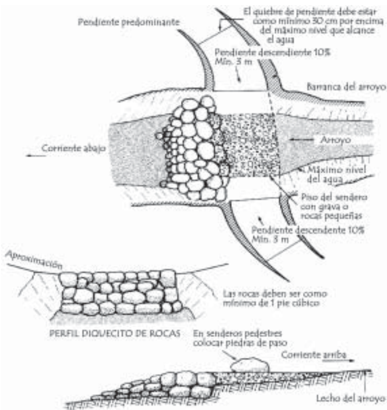
Cruce de arroyo de rocas
